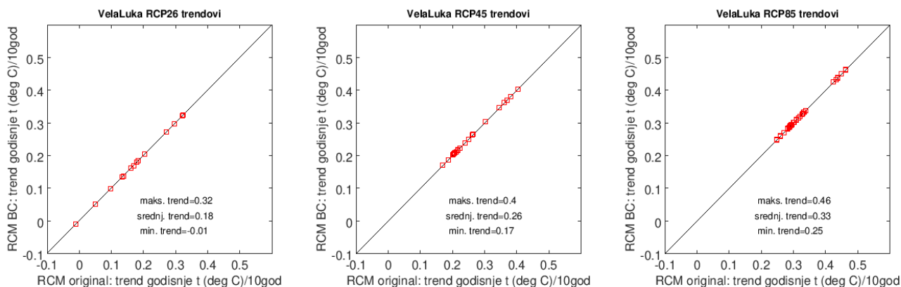
Slika 4.3.2.3 Usporedba linearnog trenda u originalnim simulacijama (x-os) te statistički obrađenim simulacijama (y-os) za razdoblje 1971. – 2070. Analizirana veličina: trend godišnje temperature zraka ( ^{\circ}\text{C}/10 god). Analiza za korištene scenarije koncentracija stakleničkih plinova RCP2.6 (lijevo), RCP4.5 (sredina) i RCP8.5 (desno). Lokacija: Vela Luka.
