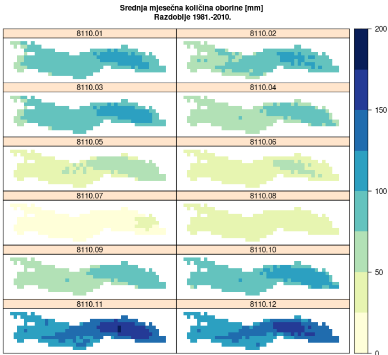
Slika 4.2.2.3 Srednje mjesečne sume količine oborine za normalu razdoblja 1981. – 2010. Paneli su naslovljeni skraćenom oznakom razdoblja (8110) i mjeseca (01,...,12).
