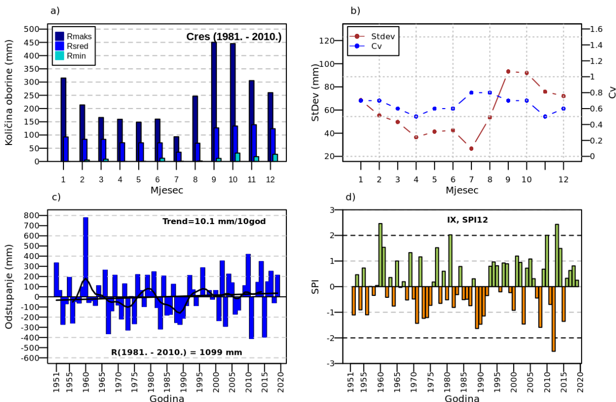
Slika 2.1.1.2 (a) Godišnji hod srednje količine oborine i (b) standardne devijacije u razdoblju 1981. – 2010. (c) Vremenski niz odstupanja godišnjih količina oborine od srednjaka, linearni trend (crna linija) i binomni klizni srednjak (crna krivulja) te (d) vrijednosti standardiziranog oborinskog indeksa (SPI) na 12-mjesečnoj skali za rujan (hidrološka godina), na postaji Cres za razdoblje 1951.–2019.
