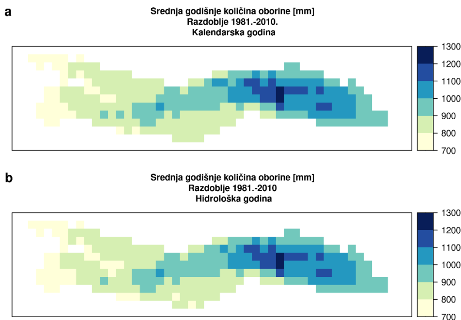
Slika 4.2.2.4 Srednja godišnja količina oborine za (a) kalendarsku i (b) hidrološku godinu. Razdoblje 1981. – 2010.
