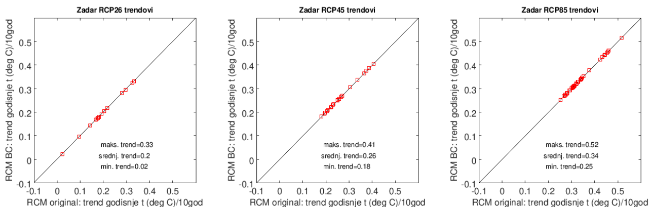
Slika 3.3.2.3 Usporedba linearnog trenda u originalnim simulacijama (x-os) te statistički obrađenim simulacijama (y-os) za razdoblje 1971. – 2070. Analizirana veličina: trend godišnje temperature zraka ( ^{\circ}\text{C}/10 god). Analiza za korištene scenarije koncentracija stakleničkih plinova RCP2.6 (lijevo), RCP4.5 (sredina) i RCP8.5 (desno). Lokacija: Zadar.
