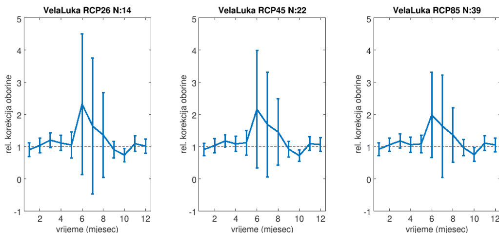
Slika 4.3.1.4 Godišnji hod relativne korekcije srednje mjesečne količine oborine (bezdimenzionalna veličina). Prikazan je srednjak i standardna devijacija mjesečnih korekcija unutar RCM ansambla za modele koji su uključeni u scenarije RCP2.6 (prvi stupac), RCP4.5 (drugi stupac) i RCP8.5 (treći stupac). Razdoblje: 1981. – 2010. Lokacija: Vela Luka.
