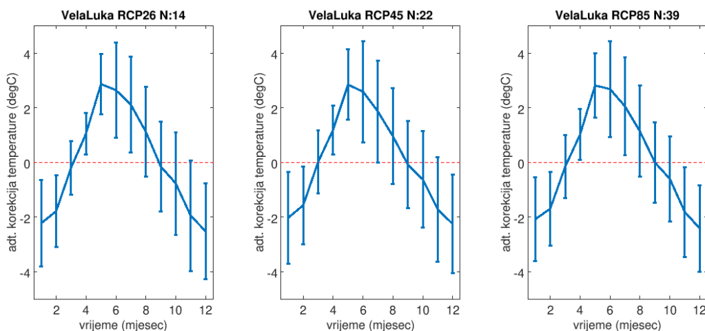
Slika 4.3.1.3 Godišnji hod aditivne korekcije srednje mjesečne temperature zraka (°C). Prikazan je srednjak i standardna devijacija mjesečnih korekcija unutar RCM ansambla za modele koji su uključeni u scenarije RCP2.6 (prvi stupac), RCP4.5 (drugi stupac) i RCP8.5 (treći stupac). Razdoblje: 1981. – 2010. Lokacija: Vela Luka.
