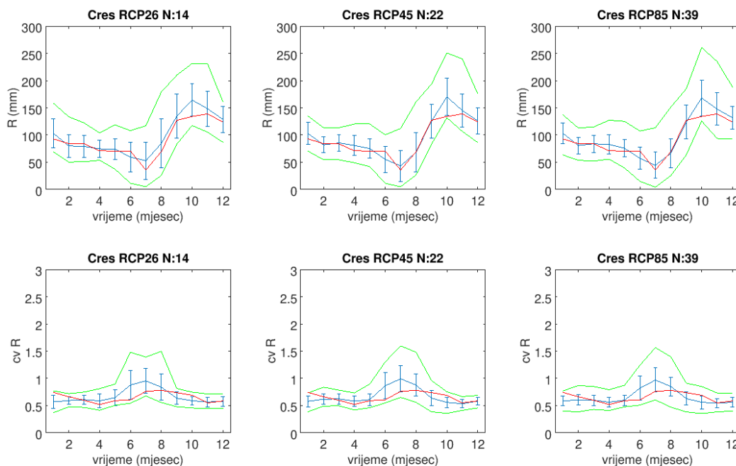
Slika 2.3.1.2 Godišnji hod srednje mjesečne količine oborine ( R , u mm; prvi red) i godišnji hod koeficijenta varijacije mjesečne količine oborine ( cvR ; drugi red). Prvi stupac: modeli uključeni u scenarij RCP2.6; drugi stupac: modeli uključeni u scenarij RCP4.5; treći stupac: modeli uključeni u scenarij RCP8.5. Plavo: srednjak i standardna devijacija unutar RCM ansambla; zeleno: raspon unutar RCM ansambla; crveno: mjerenja. Razdoblje: 1981. – 2010. Izvor: mjerenja DHMZ i izvorne simulacije regionalnih klimatskih modela. Lokacija: Cres.
