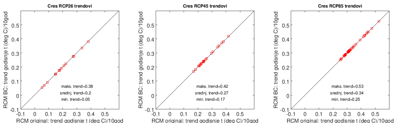
Slika 2.3.2.3 Usporedba linearnog trenda u originalnim simulacijama (x-os) te statistički obrađenim simulacijama (y-os) za razdoblje 1971. – 2070. Analizirana veličina: trend godišnje temperature zraka ( ^{\circ}\text{C}/10 god). Analiza za korištene scenarije koncentracija stakleničkih plinova RCP2.6 (lijevo), RCP4.5 (sredina) i RCP8.5 (desno). Lokacija: Cres.
