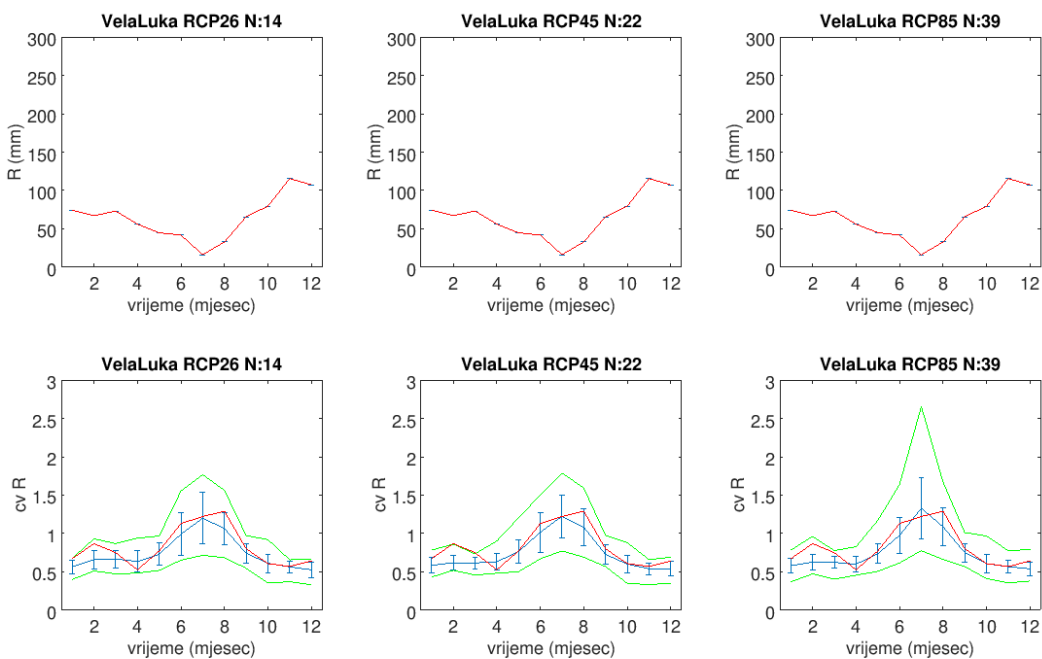
Slika 4.3.1.6 Isto kao Slika 4.3.1.2 za statistički obrađene RCM simulacije. Razdoblje: 1981. – 2010. Lokacija: Vela Luka.
